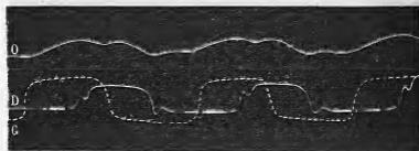
Fig. 31. — Homme galopant à droite. Foulées et réactions. On constate un empiétement d'une foulée sur l'autre, puis, une suspension du corps. — La courbe O qui correspond aux réactions montre l'effet des deux impulsions successives que les pieds impriment au corps.
